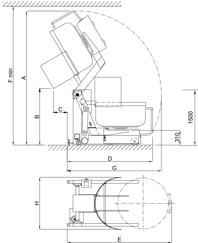
SOLLEVATORE - ROVESCIAIORE DI VASCHE / BOWL ELEVATOR
